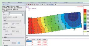
変位図と変位のコンタ表示
