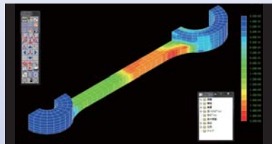
コネクティングロッド 濃染図
