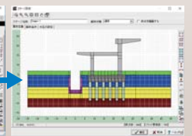
自動メッシュ分割でモデル生成
