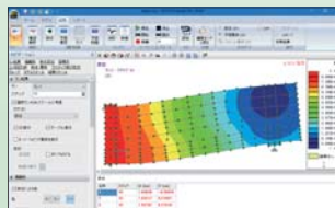
変位図と変位のコンタ表示
