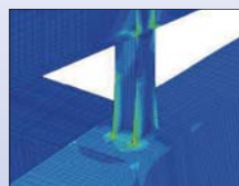
鋼上路式アーチ橋トラス・アーチ部材の応力照査
