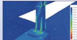
鋼上路式アーチ橋 部材の応力照査
