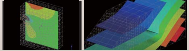
GeoFEASPost-切断面図
