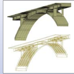
鋼上路式アーチ橋 部材の応力照査
