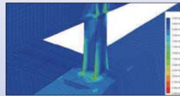
鋼上路式アーチ橋 部材の応力照査
