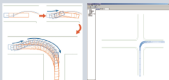
▲セミトラの後退の軌跡例 ▲メイン画面
