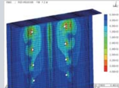
▲鋼製壁高欄の応力解析
