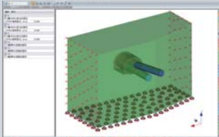
▲境界条件(弾塑性解析)
