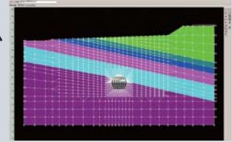
▲トンネル掘削解析-プリプロセス
