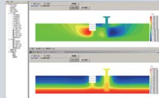
▲土留め掘削解析結果(X方向コンタ図)
