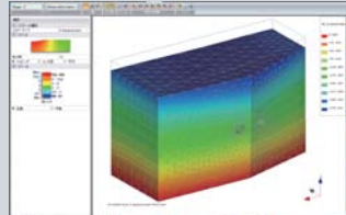
▲変位図(弾塑性解析)
