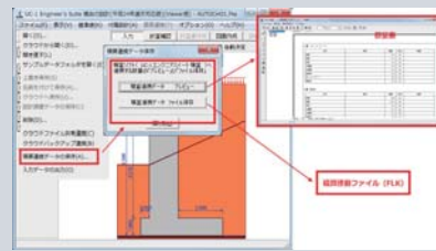
▲橋台の設計・3D配筋から数量を連動
