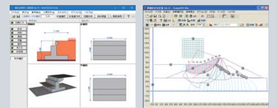
▲橋台の設計・3D配筋 Ver.15
