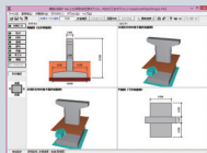
▲橋脚の設計・3D配筋
