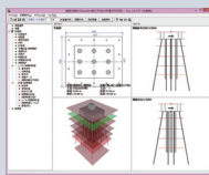
▲基礎の設計・3D配筋
