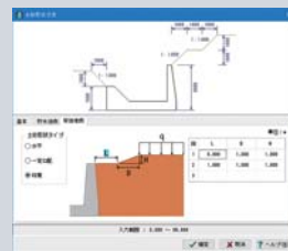
▲土砂形状入力画面
