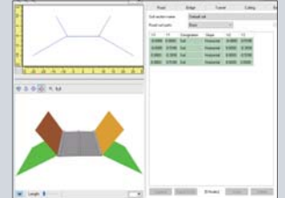
▲土工断面定義画面 / 自動的にデフォルトの土工断面を生成
