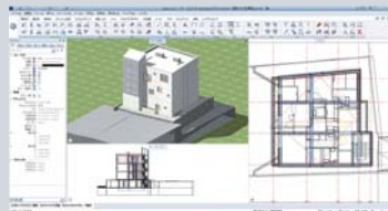
▲Allplan
