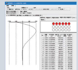
▲せん断耐力算出詳細表
