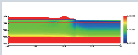
▲液化化安全率 (FL) の分布図
