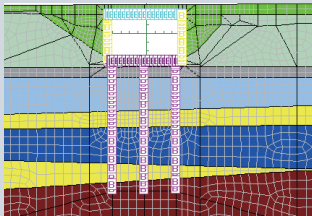
▲応答震度法によるボックスカルバートの検討例
