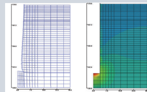
▲最終掘削時の変形、変位コンタ図
