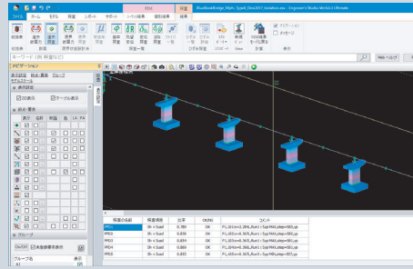
▲免震支承を設置した連続橋の動的照査に関するサンプルデータ
