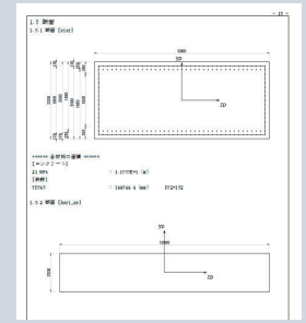
▲レポート出力で断面に主軸 zp-ypを明示
