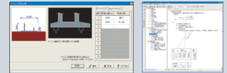
▲フーチング照査位置の入力画面 ▲計算書プレビュー
