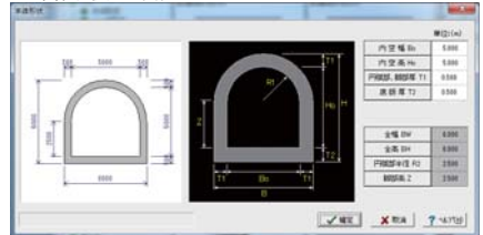
▼結果確認画面
