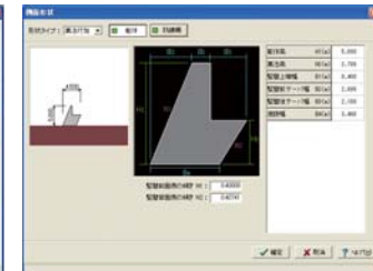
▼重力式擁壁-裏法付加
