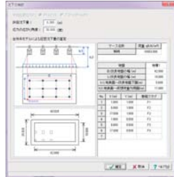
▼沈下の検討入力
