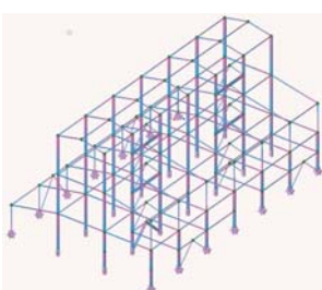
▼Engineer's Studio®に変換したデータ
