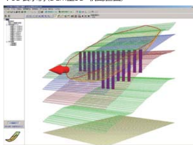
▼3D表示例 (DEM型3D: 杭配置図)
