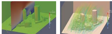
▲中目黒駅周辺のメッシュと風速分布図(コンター/ベクトル)
