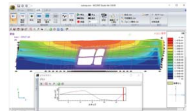
▼地盤と構造物の一体解析結果
