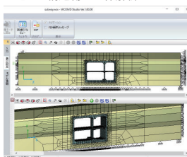
▼地盤と構造物の一体解析モデル
