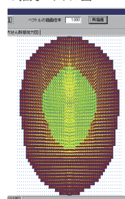
▼推力ベクトル図
