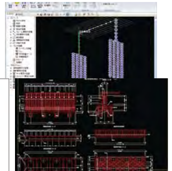
▲橋台壁配筋図
