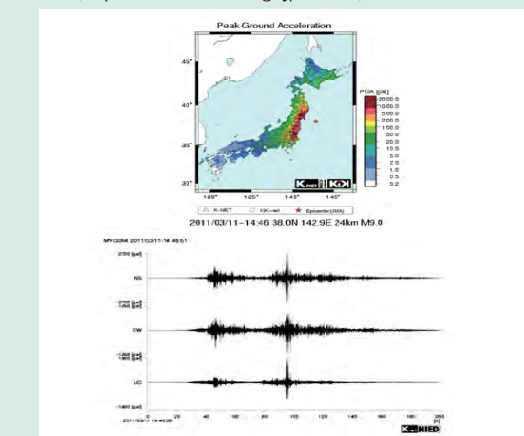
強震観測網(K-NET, KiK-net)により観測された地表での最大化速度分布(左)とK-NET築館(MYG004)観測点の強震動波形(右)(防災科学技術研究所HP)
