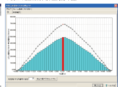
▼杭工の設計計算(抑止力分布図)
