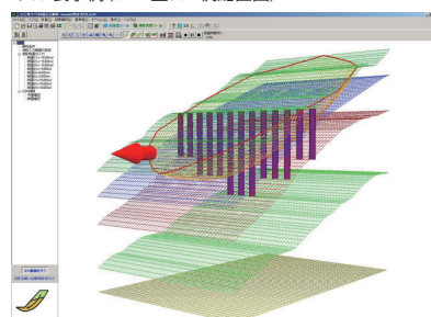
▼3D表示例(DEM型3D: 杭配置図)
