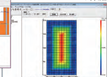
▼等水位線図
