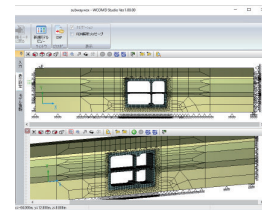
▼地盤と構造物の一体解析モデル
