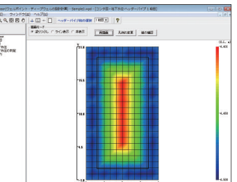
▼等水位線図
