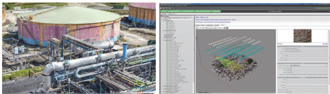
▲ContextCapture：リアリティメッシュ(写真テクスチャ付3Dモデル)により、現実のコンテキストを正確に反映(左)/写真から空中三角測量を自動実行可能(右)
