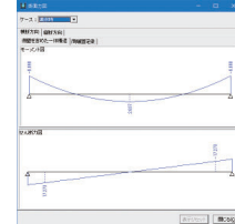
▼断面力図
