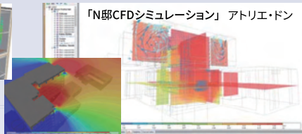
「N邸CFDシミュレーション」アトリエ・ドン
