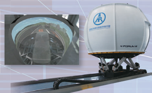
8DOF 交通安全シミュレータ
