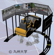
6DOF0.7G対応モーション シミュレータシステム
