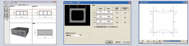
▲メイン画面(3連BOX) ▲単鉄筋構造の配筋画面 ▲結果確認(断面力図)
