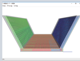
▲3D配筋ビューア (U型擁壁Bタイプ)
