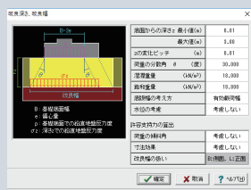
▲改良深さ、改良幅設定画面
