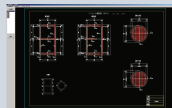
▲2D配筋機能
