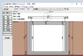
▲メイン画面 (蓋付きU型擁壁)
