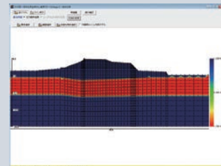
▲河川堤防(液状化安全率(FL))の結果
