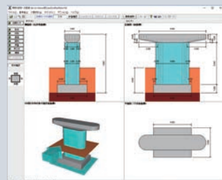
▲橋脚の設計・3D配筋
