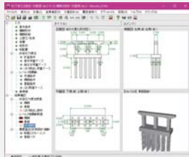
▲ラーメン橋脚の設計・3D配筋
