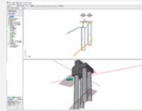
▲深礎フレームの設計・3D配筋
