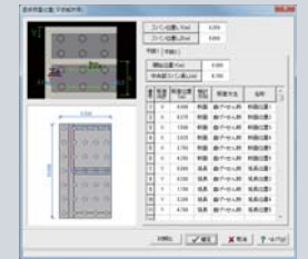
▲平板解析用底版照査位置入力
