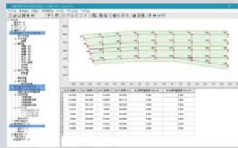
▲作用の種類
