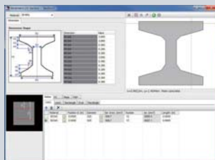
▲入力画面の例(せん断関連)
