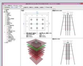
▲基礎の設計・3D配筋 (部分係数法・H29道示対応)
