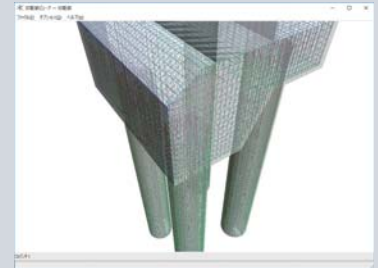
▲3D配筋
