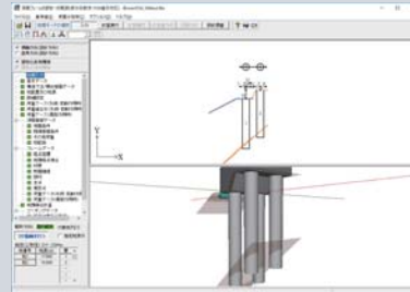
▲メイン画面(杭基礎)
