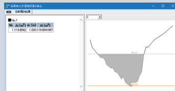
▲計画捕捉量の断面結果
