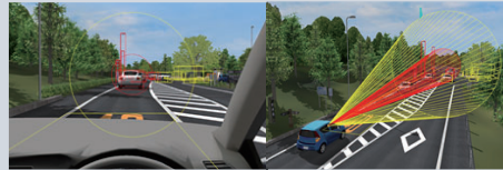
▲オブジェクト検出 検出範囲と交差しているオブジェクトを検出。
