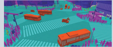
▲レンダリング処理カスタマイズ オブジェクト種別、深度、速度、加速度の情報等を元に色付け。
