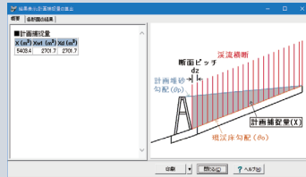
▲計画捕捉量の概算
