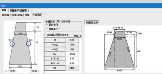
▲非越流部の計算設定
