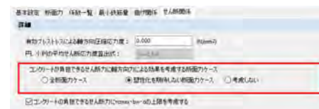
▲軸方向力による効果を考慮する断面力ケース
