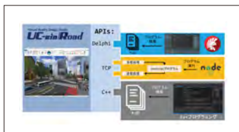
▲C++API構成
