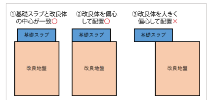
▲改良体の偏心配置
