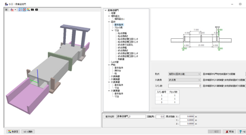
▲柔構造樋門—入力画面
