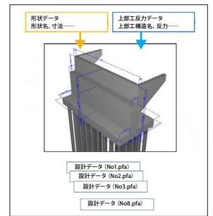
▲CSVファイルからの自動生成機能
