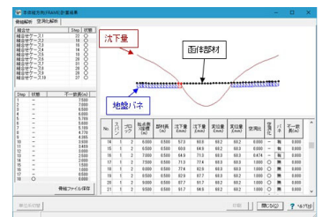
▲空洞化解析結果画面
