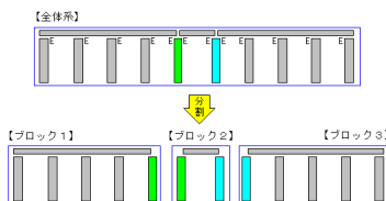
▲ブロック単位のイメージ
