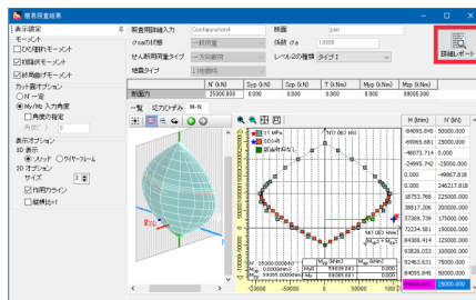
▲M-N相互作用図と「詳細レポート」ボタン
