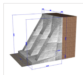
▲逆L型支え壁式擁壁
