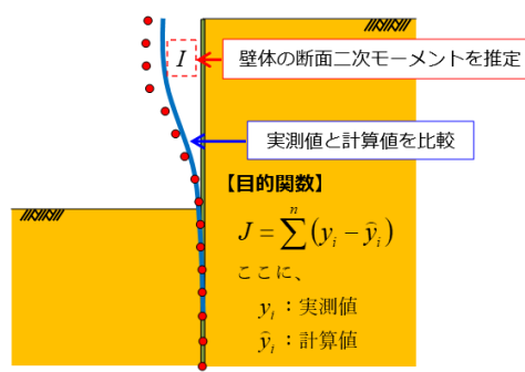
▲逆解析による壁体剛性（断面二次モーメント）の推定
