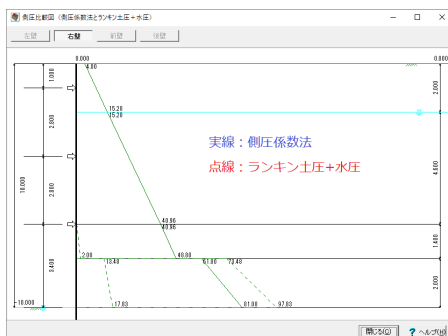
▲側圧比較図（[結果確認]画面）
