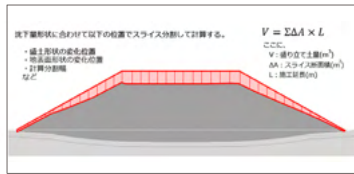
▲盛り立て土量の算出
