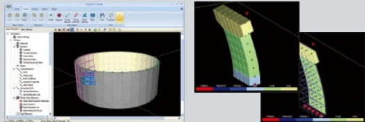
▲メイン画面 ▲平板の変形とひずみ損傷判定結果
